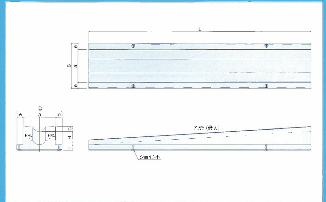
SE インバート 寸法図
