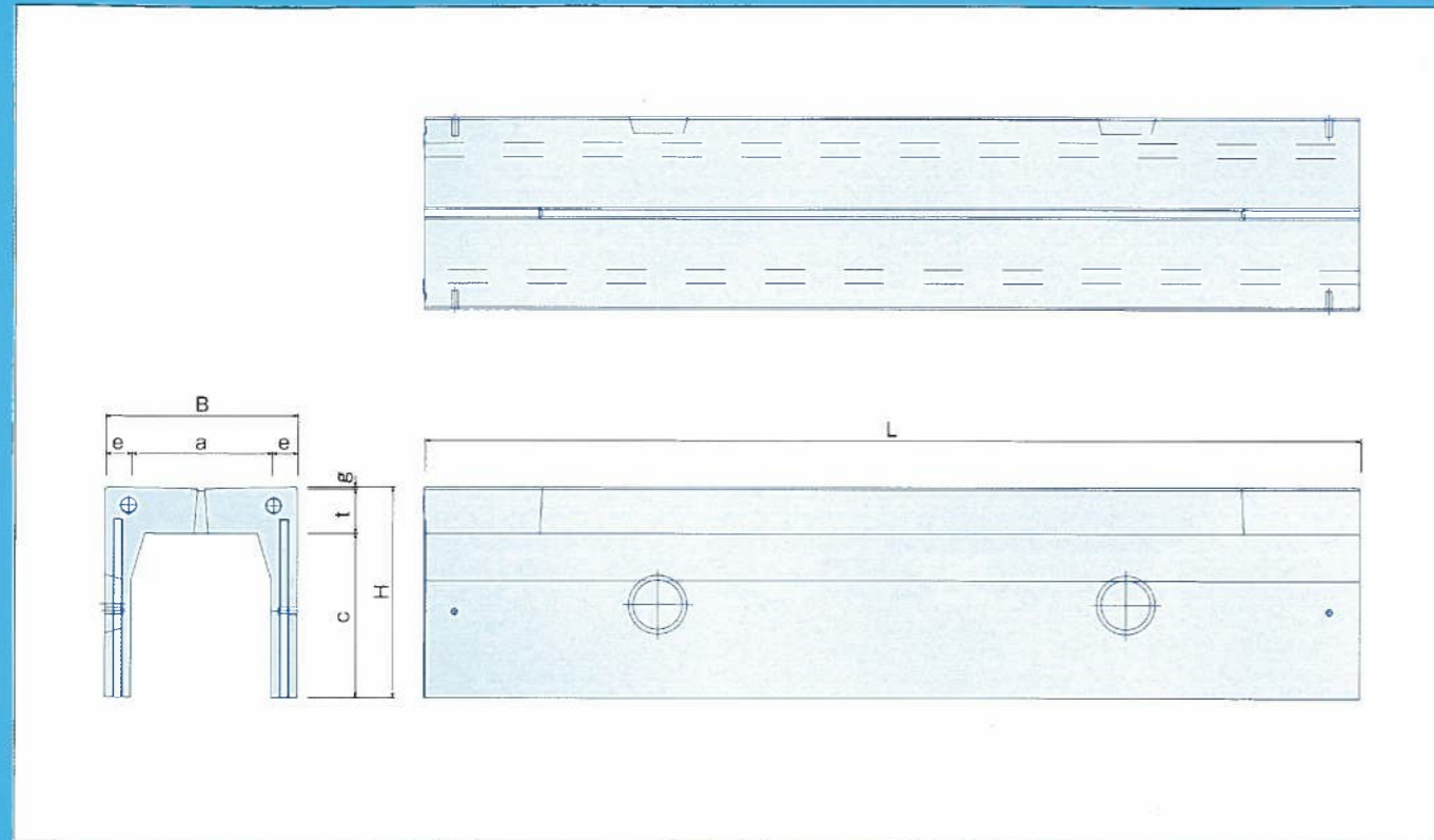
SE-K 寸法図
