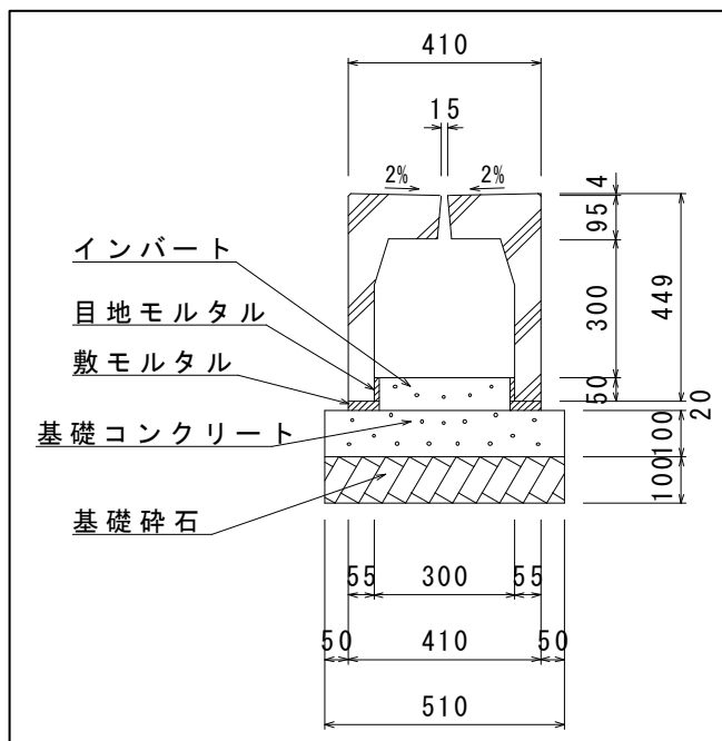
施工標準図
